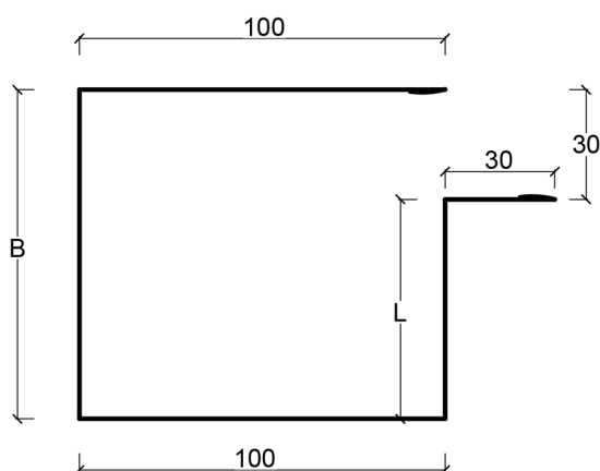
CANALETA DE LLUVIA PARA TR5
