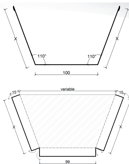
CANALETA DE LLUVIA PARA COBERTURA CURVA
